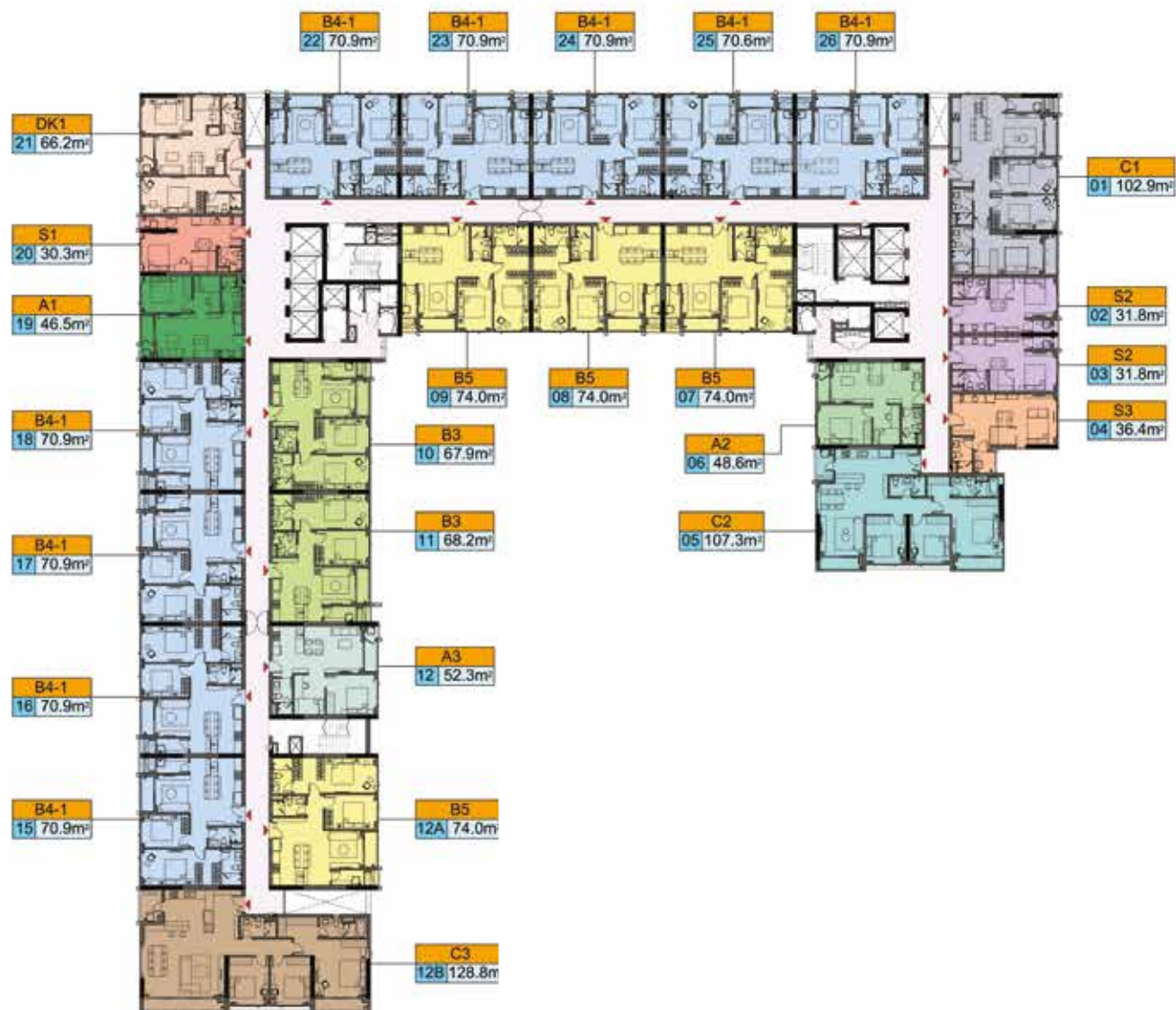
Mặt bằng tầng 7 - 24
