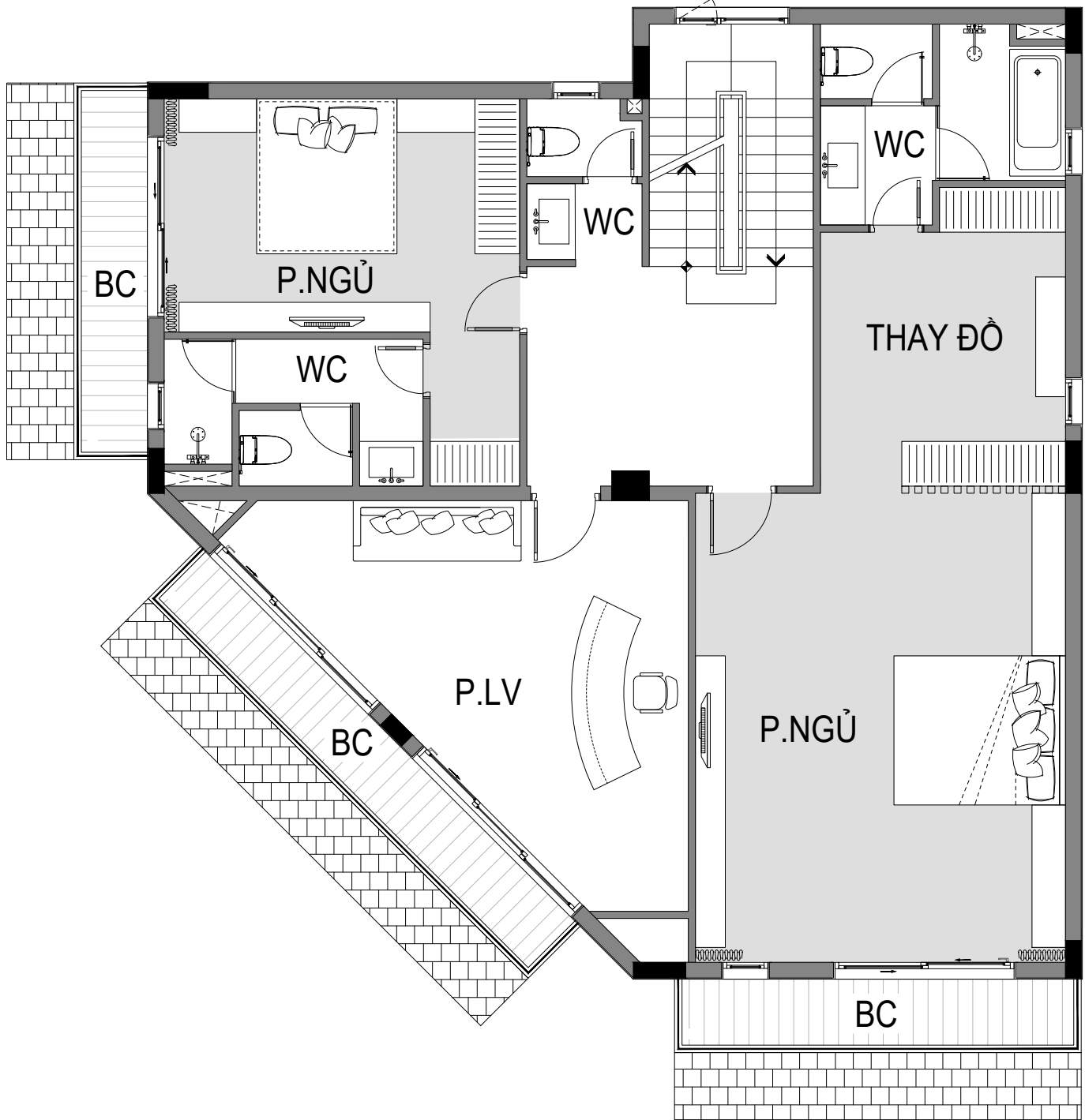
MẶT BẰNG TẦNG 3
