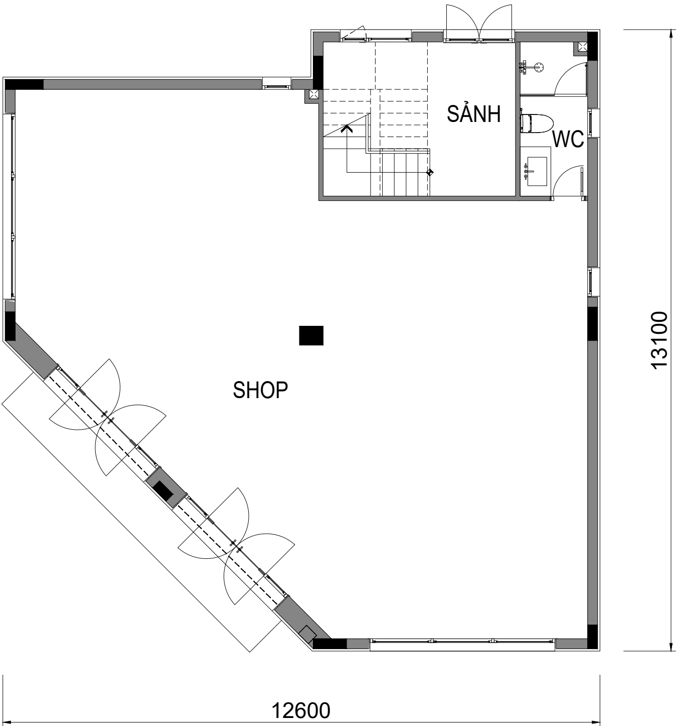
MẶT BẰNG TẦNG 1
