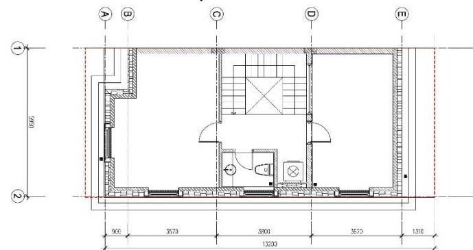
MẶT BẰNG TẦNG 5
