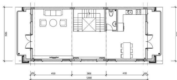
MẶT BẰNG TẦNG 2
