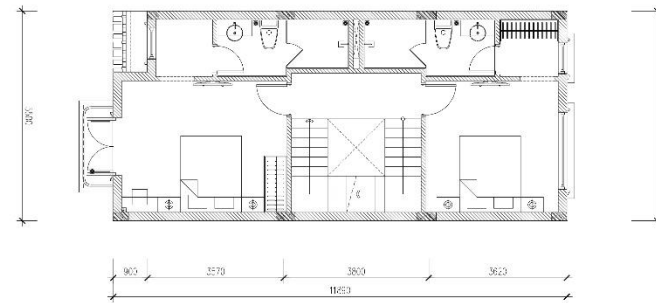
MẶT BẰNG TẦNG 4
