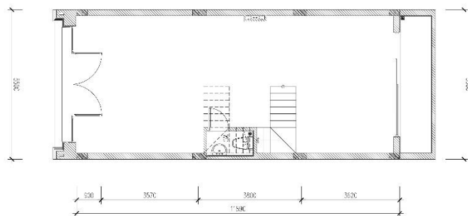
MẶT BẰNG TẦNG 1
