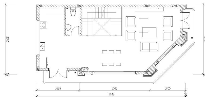
MẶT BẰNG TẦNG 2
