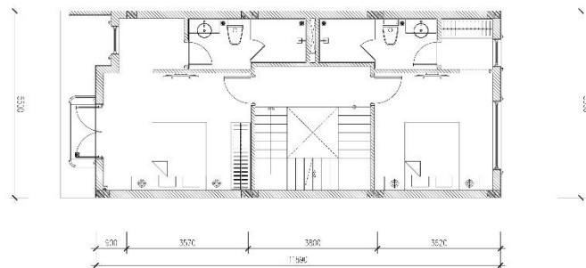
MẶT BẰNG TẦNG 3
