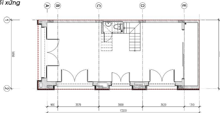
MẶT BẰNG TẦNG 1
