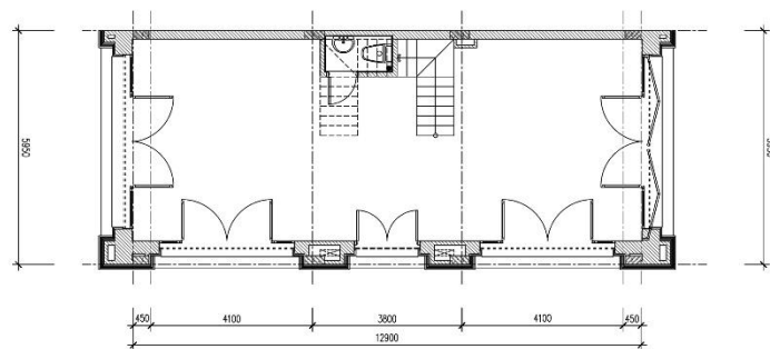
MẶT BẰNG TẦNG 1
