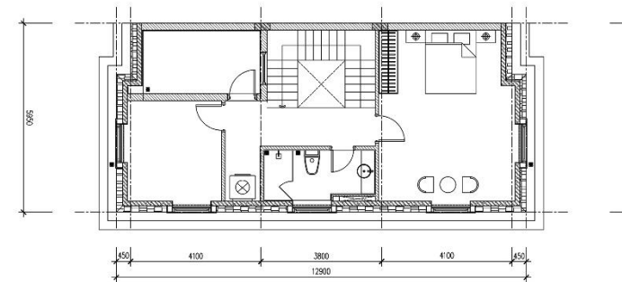
MẶT BẰNG TẦNG 4
