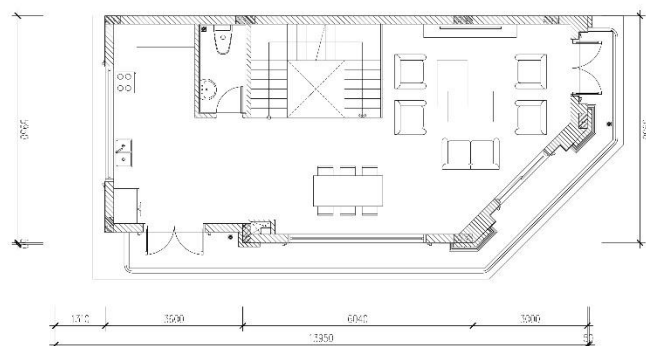
MẶT BẰNG TẦNG 2
