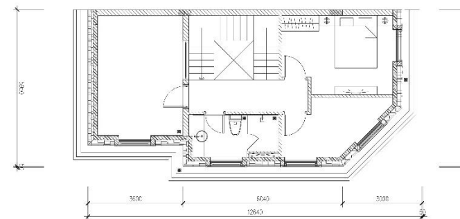
MẶT BẰNG TẦNG 4
