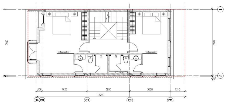
MẶT BẰNG TẦNG 3
