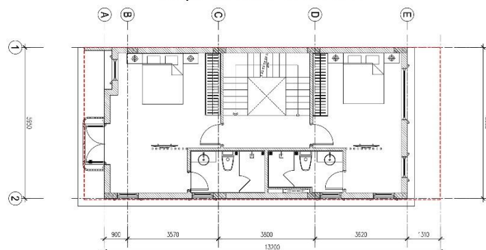
MẶT BẰNG TẦNG 3
