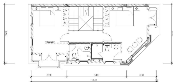
MẶT BẰNG TẦNG 3
