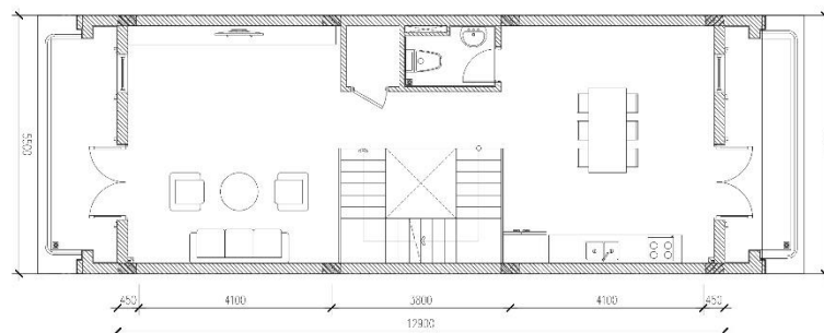
MẶT BẰNG TẦNG 2
