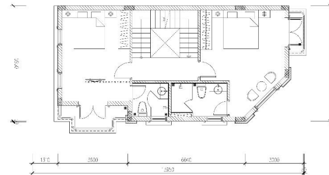
MẶT BẰNG TẦNG 4
