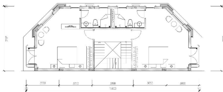
MẶT BẰNG TẦNG 3
