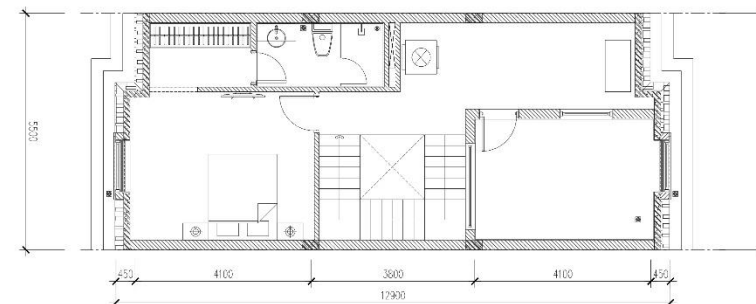
MẶT BẰNG TẦNG 4
