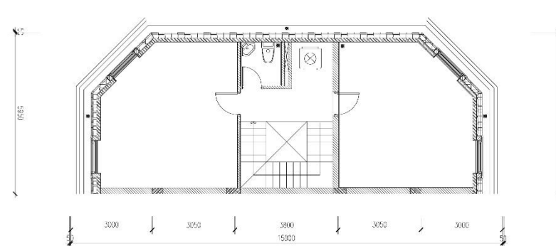
MẶT BẰNG TẦNG 5
