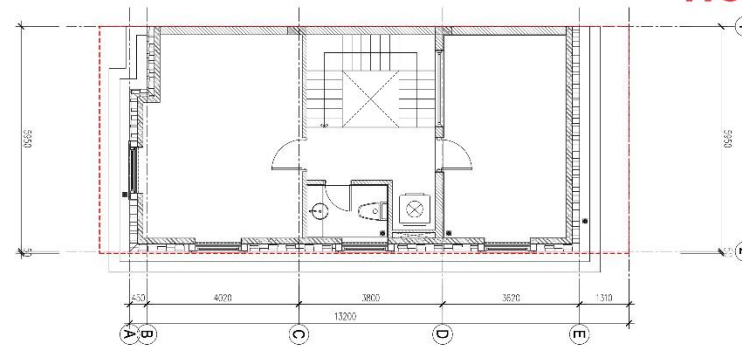
MẶT BẰNG TẦNG 4
