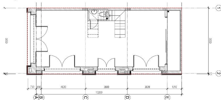
MẶT BẰNG TẦNG 1
