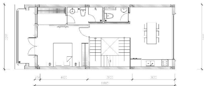
MẶT BẰNG TẦNG 2
