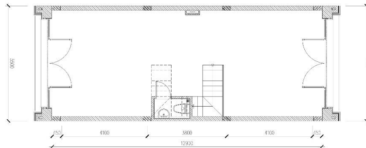
MẶT BẰNG TẦNG 1
