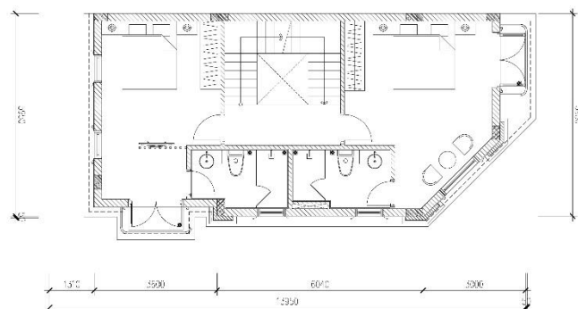
MẶT BẰNG TẦNG 3
