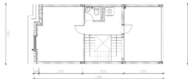
MẶT BẰNG TẦNG 4
