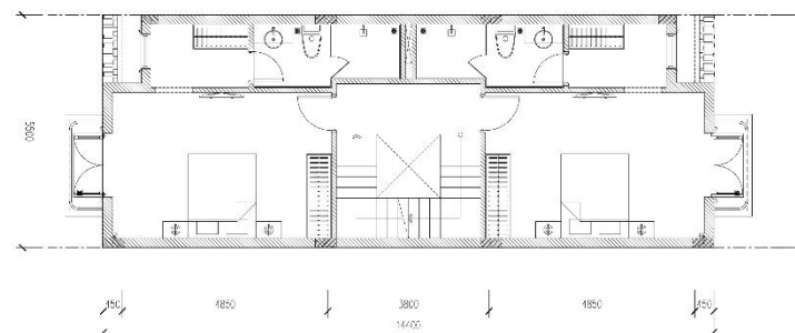
MẶT BẰNG TẦNG 4
