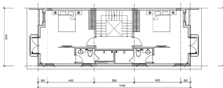
MẶT BẰNG TẦNG 3
