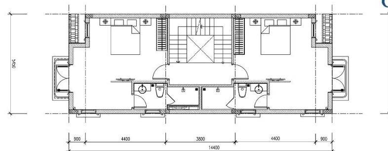
MẶT BẰNG TẦNG 4
