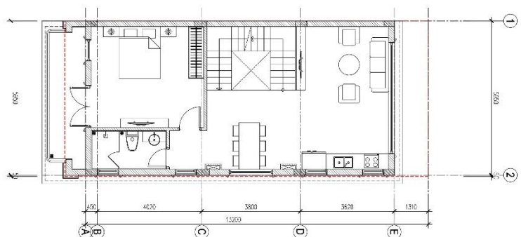
MẶT BẰNG TẦNG 2
