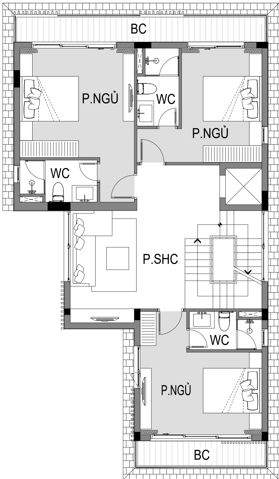
MẶT BẰNG TẦNG 2
