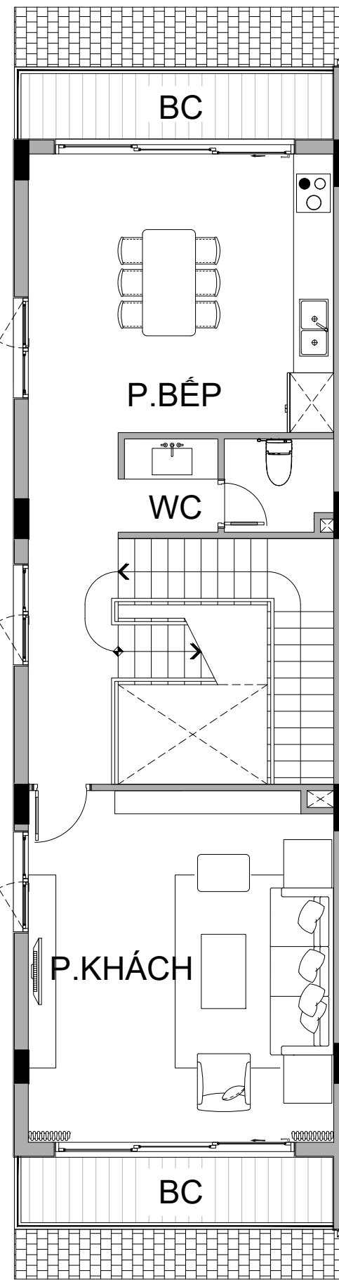
MẶT BẰNG TẦNG 2
