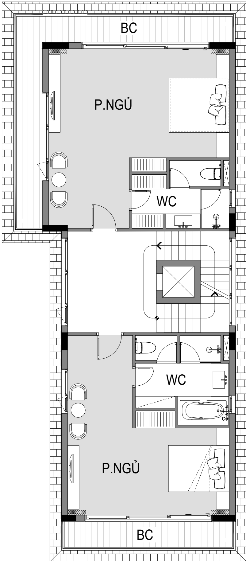
MẶT BẰNG TẦNG 3
