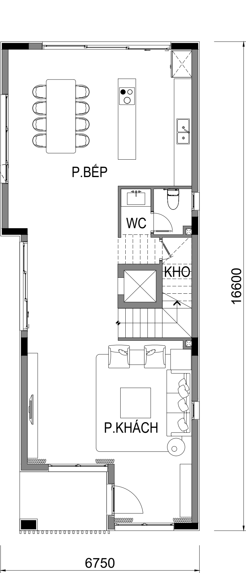
MẶT BẰNG TẦNG 1
