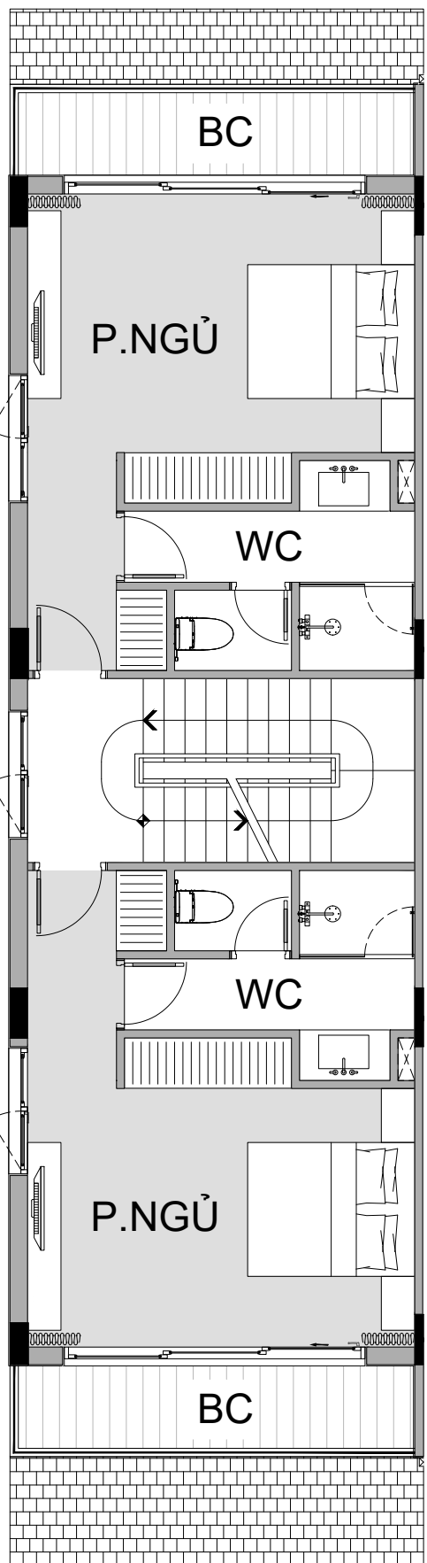
MẶT BẰNG TẦNG 4
