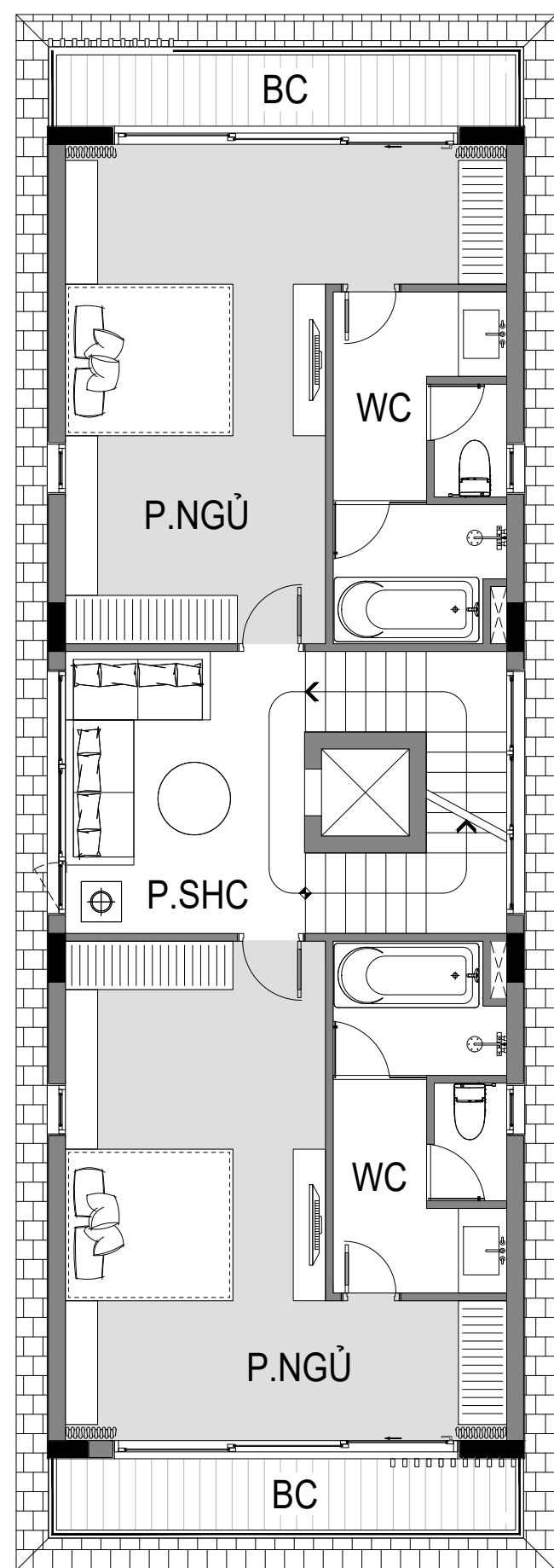
MẶT BẰNG TẦNG 2
