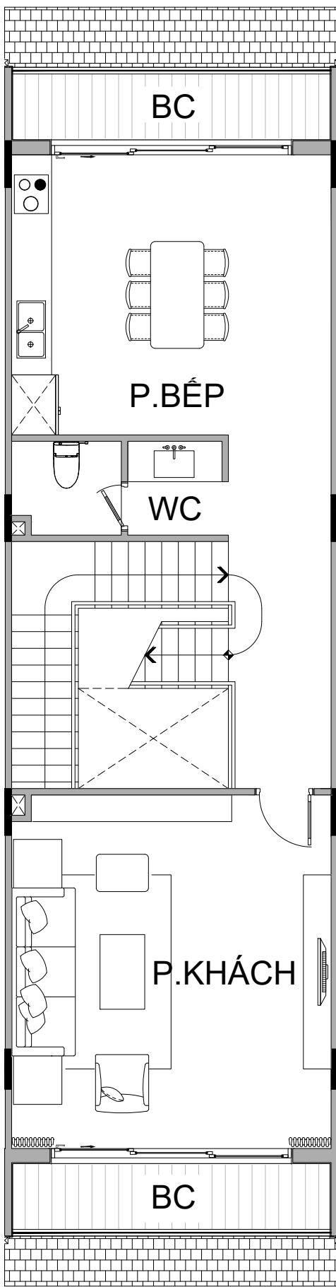
MẶT BẰNG TẦNG 2
