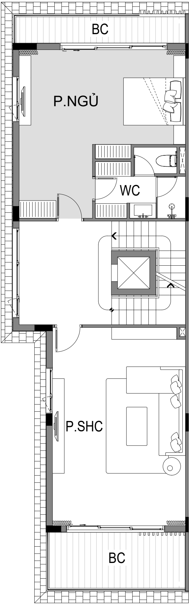
MẶT BẰNG TẦNG 2
