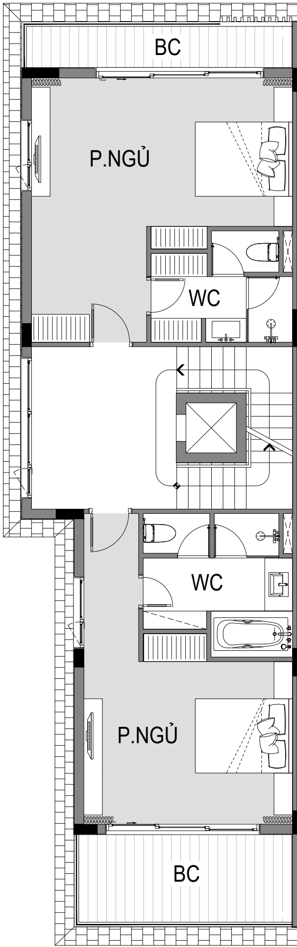
MẶT BẰNG TẦNG 3
