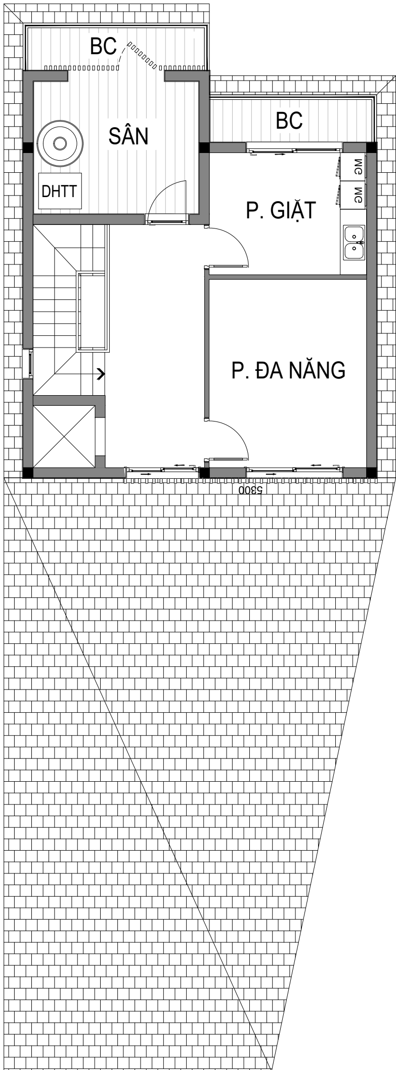
MẶT BẰNG TẦNG 4
