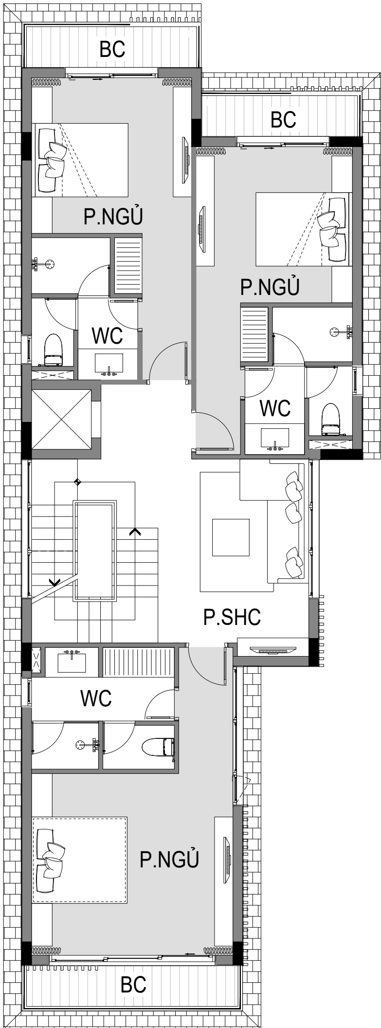
MẶT BẰNG TẦNG 2
