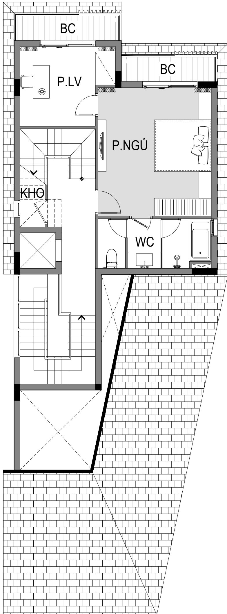
MẶT BẰNG TẦNG 3
