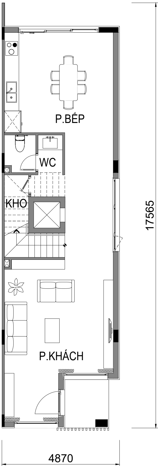
MẶT BẰNG TẦNG 1
