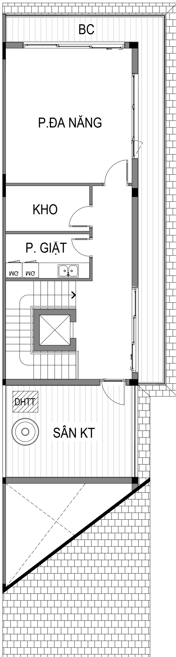
MẶT BẰNG TẦNG 4
