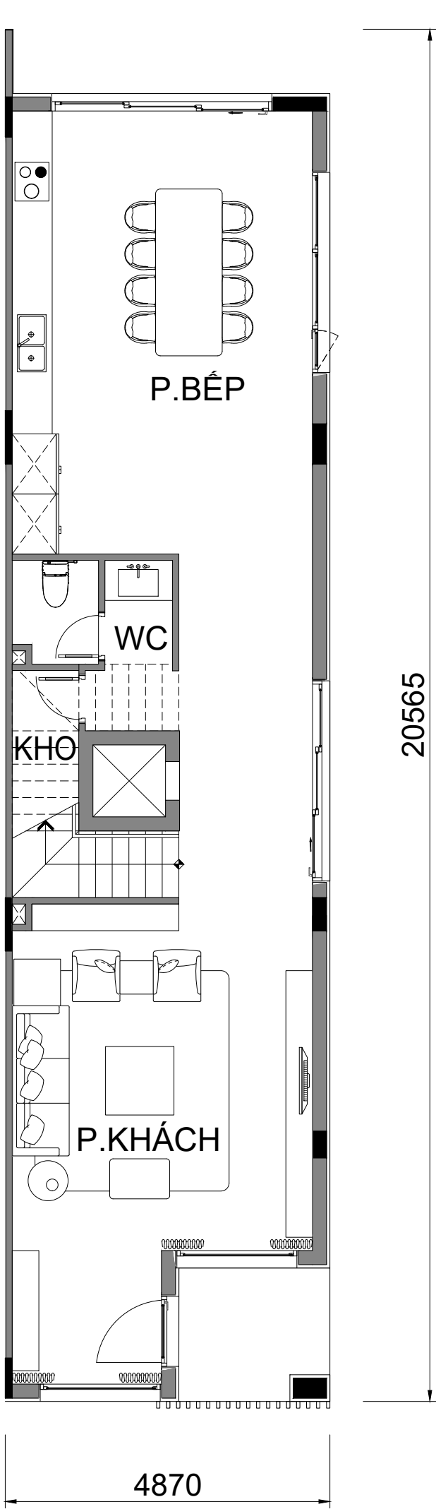
MẶT BẰNG TẦNG 1
