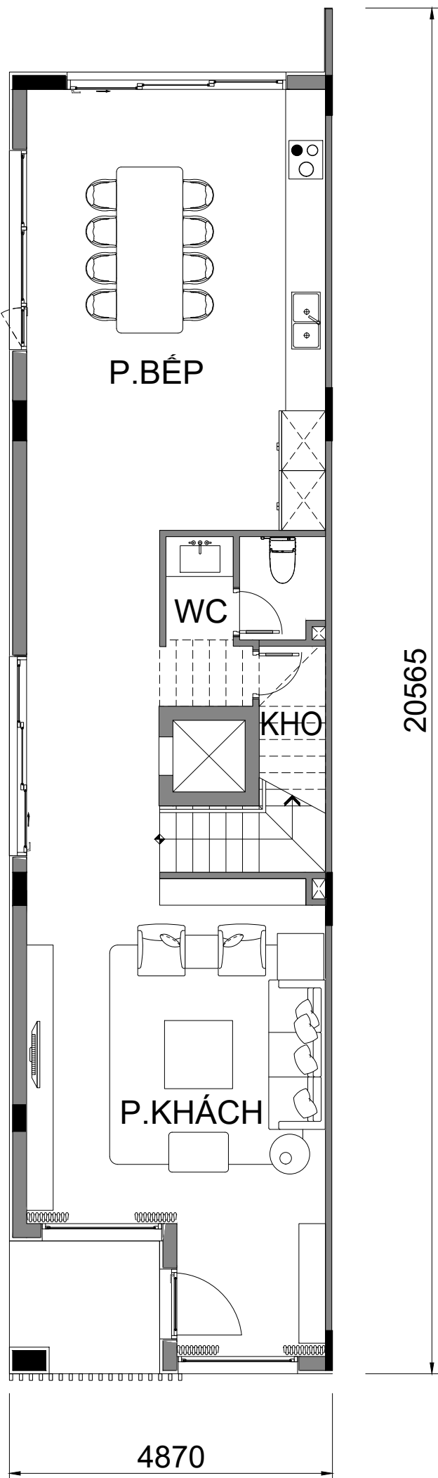
MẶT BẰNG TẦNG 1
