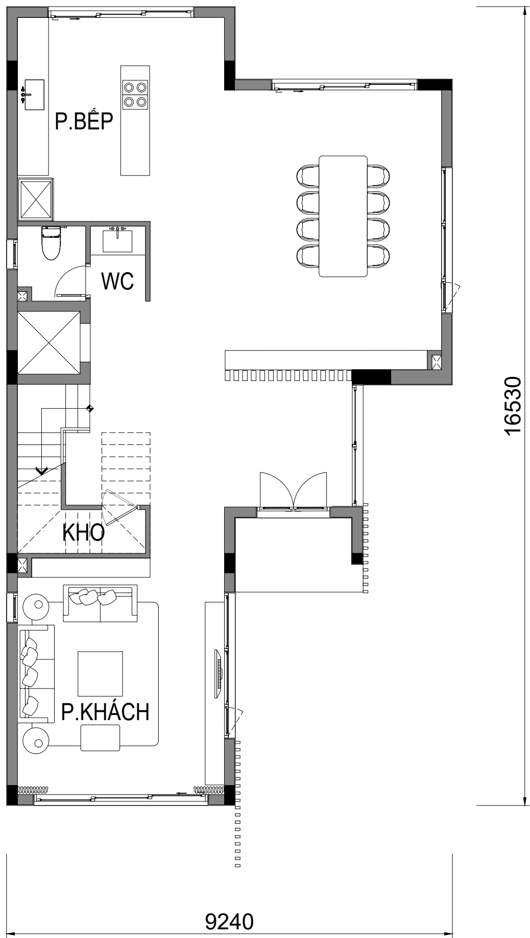
MẶT BẰNG TẦNG 1
