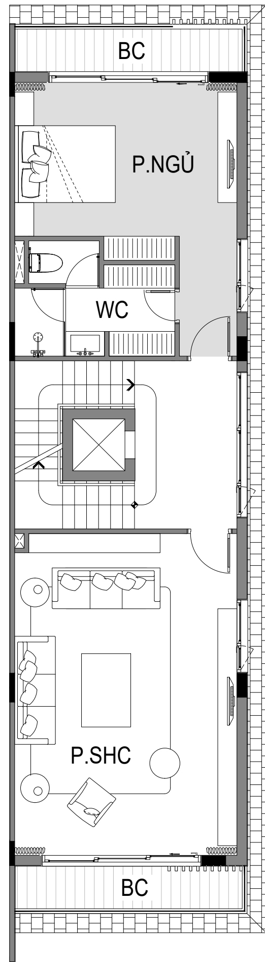
MẶT BẰNG TẦNG 2
