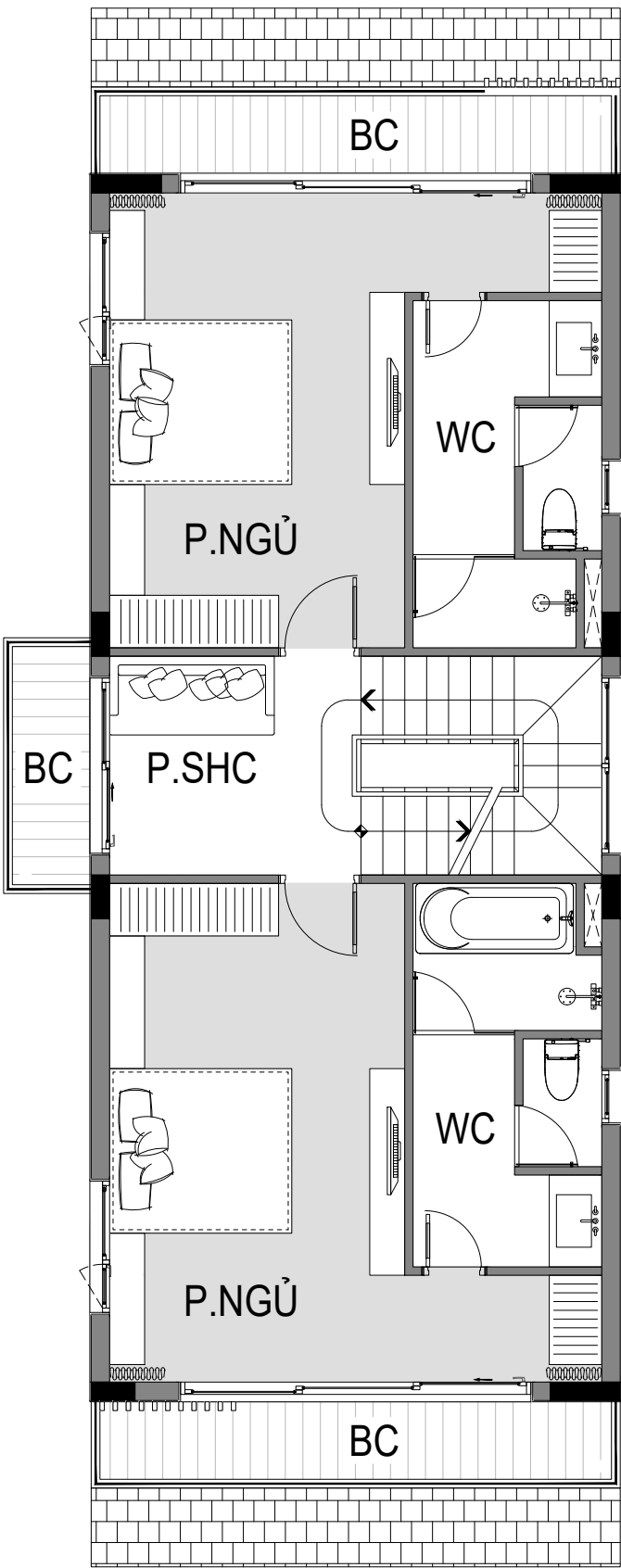
MẶT BẰNG TẦNG 3
