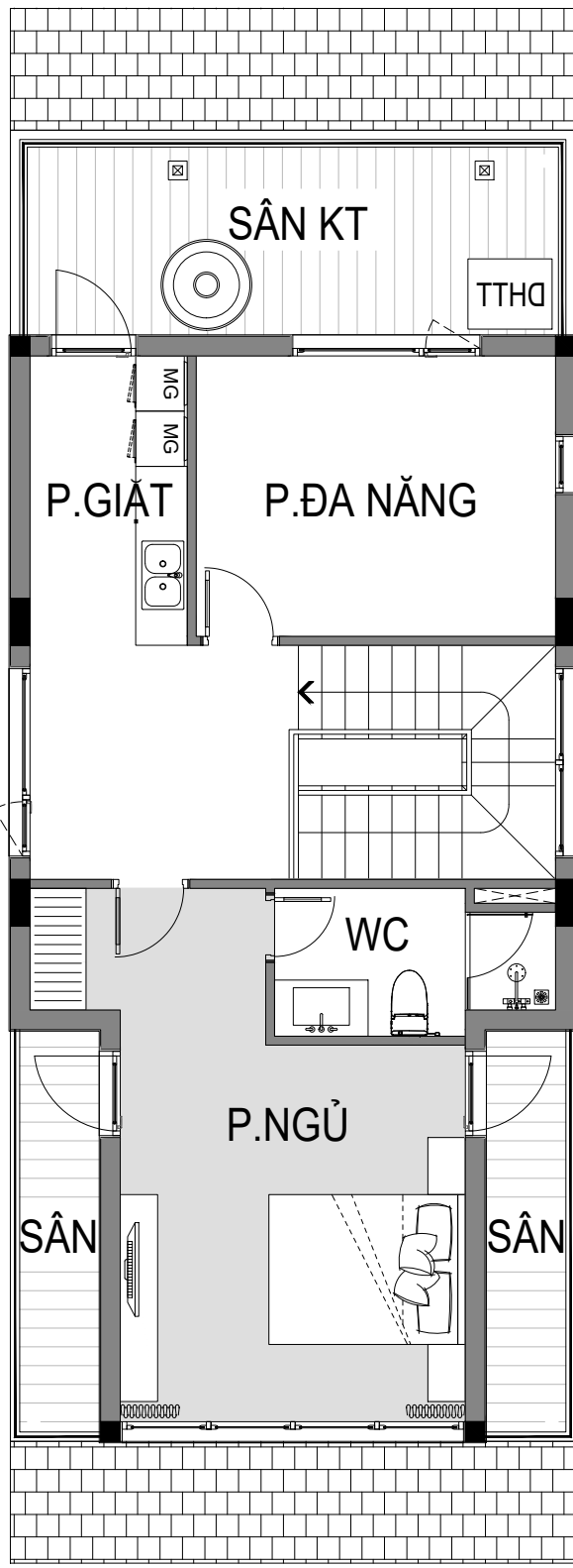
MẶT BẰNG TẦNG 4
