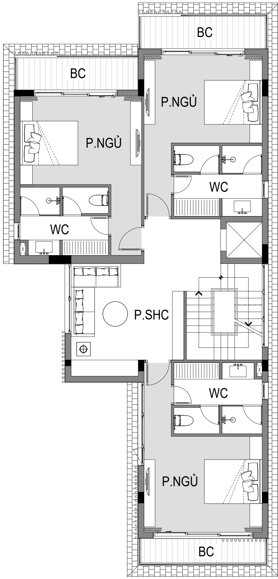
MẶT BẰNG TẦNG 2
