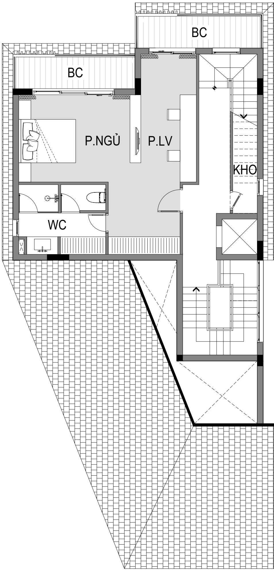
MẶT BẰNG TẦNG 3
