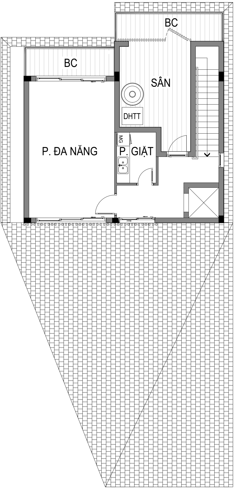
MẶT BẰNG TẦNG 4
